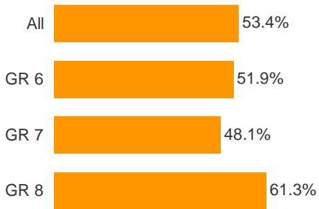
MAP Math 2018-19
