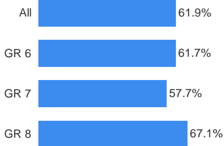
MAP Math 2018-19
